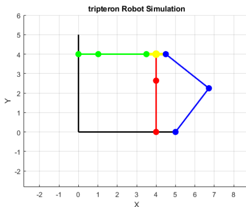
รูปที่ X ภาพการ simulation เมื่อ t = 6 สีแดง = X-leg สีเขียว = Y-leg สีฟ้า = Z-leg สีเหลือง = จุด EE
